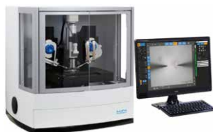
▲マイクロマニピュレーター アクシクプロ
