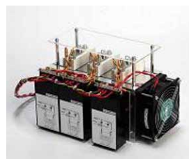
空冷サイリスタスタック 半導体製造空冷装置用制御装置付
