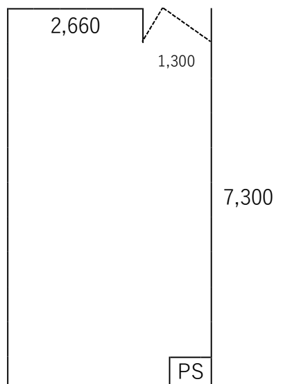
＜参考＞ 207 号室(オフィス仕様)の配置図
