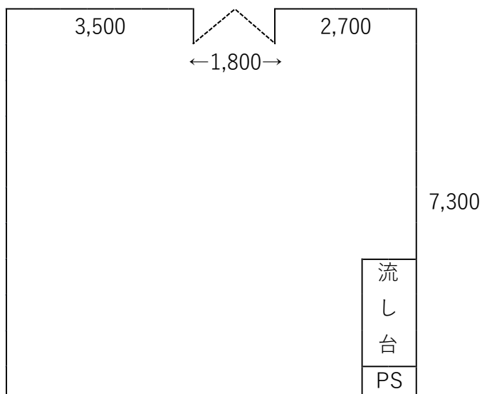
＜参考＞ 302 号室(ラボ仕様)の配置図
