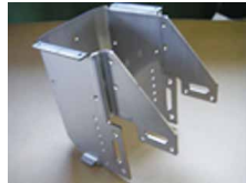
ブラケット/SUS304 2B/t2.0
